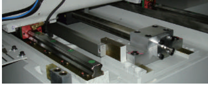
棒型 線性馬達
