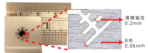
微細紡口錫鋼模具
