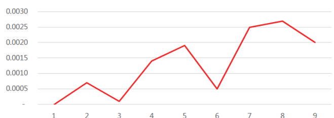
Y軸節距精度： 0.0\mu\text{m}\sim 2.7\mu\text{m}
